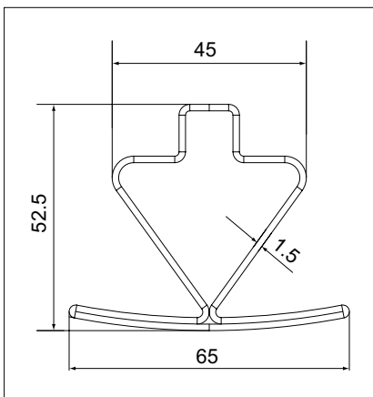
Bild 3: Querschnitt LEO 2
