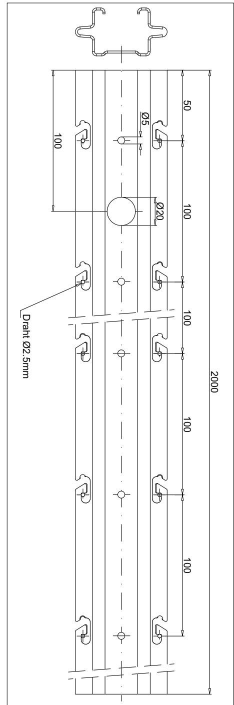
Bild 2: REMAG-Weinbergpfosten GEMINI S (Systemskizze)
