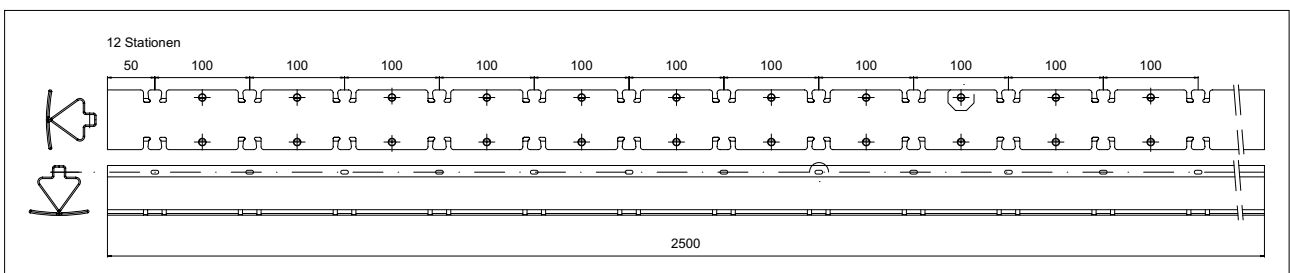
Bild 4: REMAG-Endpfosten LEO 2 (Systemskizze)
