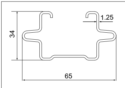
Bild 1: Querschnitt GEMINI N
