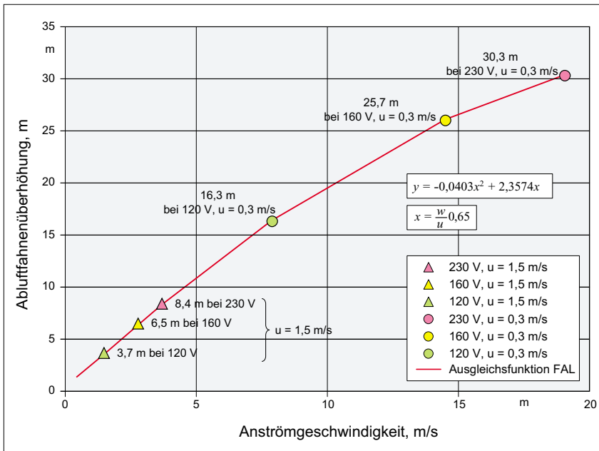
Bild 11: Abluffhohenüberhöhungen für ausgewählte Betriebsspannungen bei zwei Geschwindigkeiten im Niedrigwindbereich mit eingebautem Nachleitrad im 230 und 160 V – Abluftkaminsystem und bei 230 V Betriebsspannung und 10 Pa Widerstand des angenommenen Lüftungssystems
